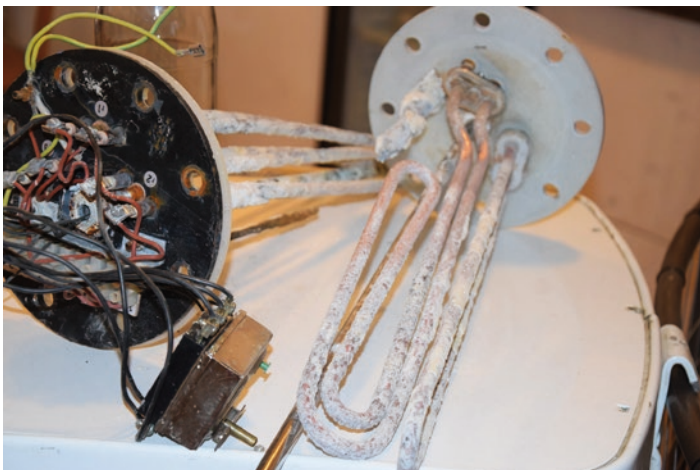
Verkalkte Boiler-Heizstäbe
